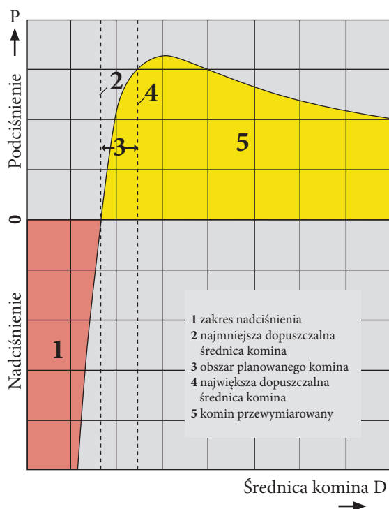
Rys. 30. Doboru rozmiaru kominu dla warunków panujących w przewodzie kominowym, z ciągiem naturalnym.
