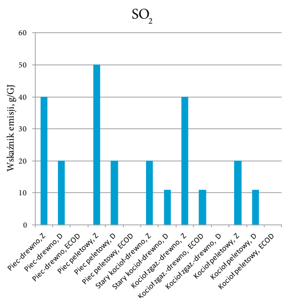
Rys. 18. Emisja zanieczyszczeń ze spalania drewna i pellet w różnych urządzeniach grzewczych Z – stara technika, D – nowa technika, ECOD – wymogi dyrektywy ErP
