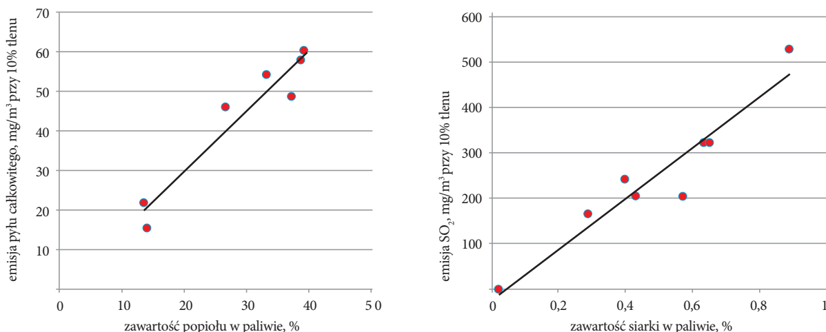
Rys. 27. Wpływ zawartości popiołu i siarki w węglu spalonym w kotle z automatycznym załadunkiem paliwa na emisję pyłu oraz SO 2 (mg/m³ przy 10% O 2 w spalinach)
