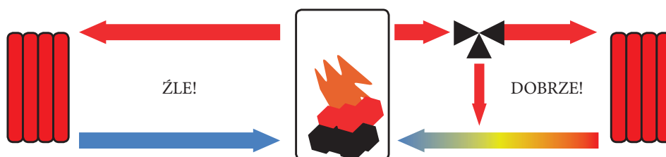
Rys. 34. Zastosowanie zaworu mieszającego
