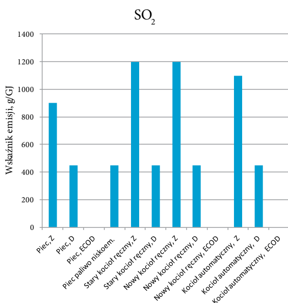
Rys. 17. Emisja zanieczyszczeń ze spalania węgla w różnych urządzeniach grzewczych Z – stara technika, D – nowa technika, ECOD – wymogi dyrektywy ErP
