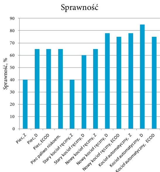
Rys. 19. Sprawność spalania węgla i drewna w różnych urządzeniach grzewczych Z – stara technika, D – nowa technika, ECOD – wymogi dyrektywy ErP
