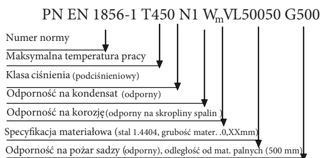
Rys. 32. Sposób znakowania elementów wkładu kominowego
