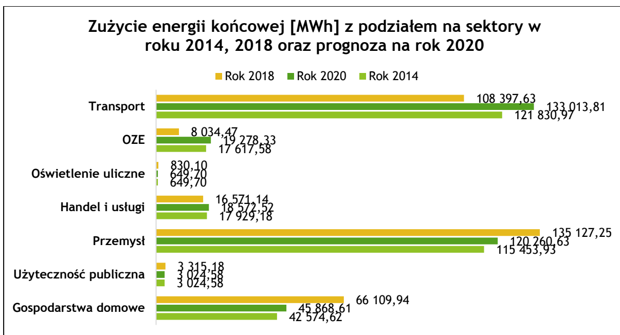
Rysunek 15. Graficzne zestawienie zużycia energii końcowej na terenie Gminy Mszczonów w ujęciu sektorowym w roku bazowym, kontrolnym oraz prognoza na rok 2020
